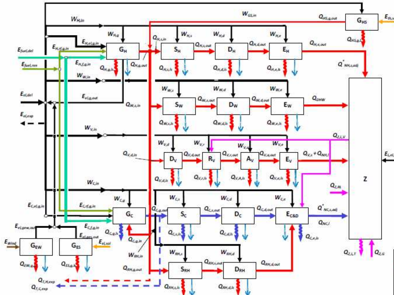
Figura 11 – Schematizzazione dell'impianto termico nella sua configurazione più generale
